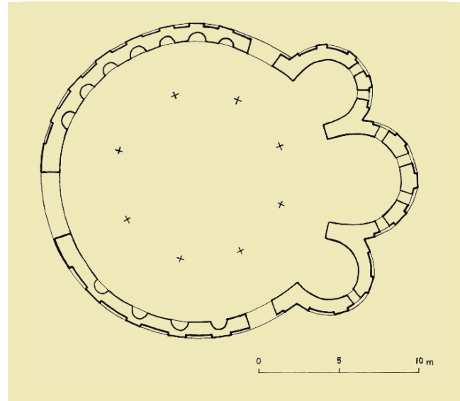
2. Tlocrt rotunde Sv. Trojstva u Zadru (izvor: VEŽIĆ, P., 2002.)
